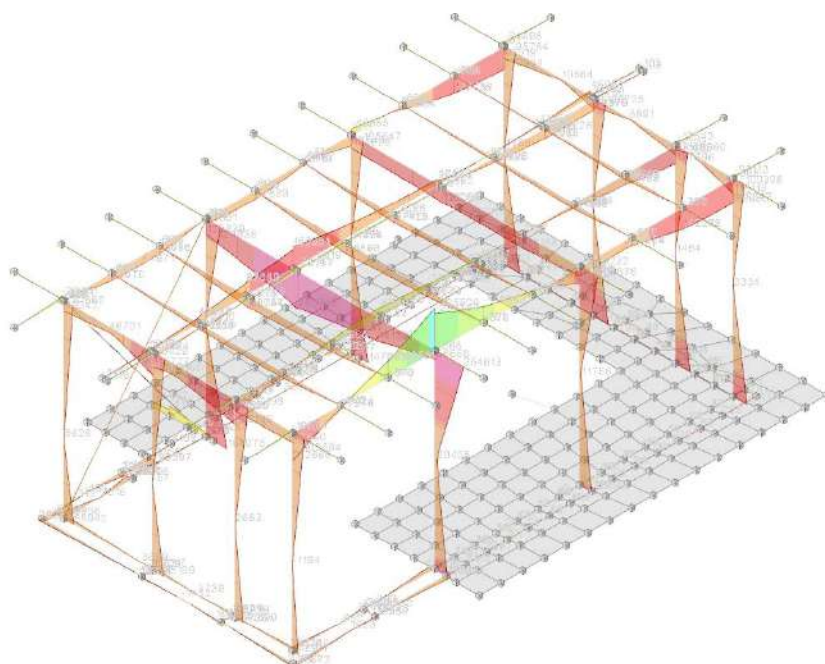
sollecitazioni aste M3 massime
