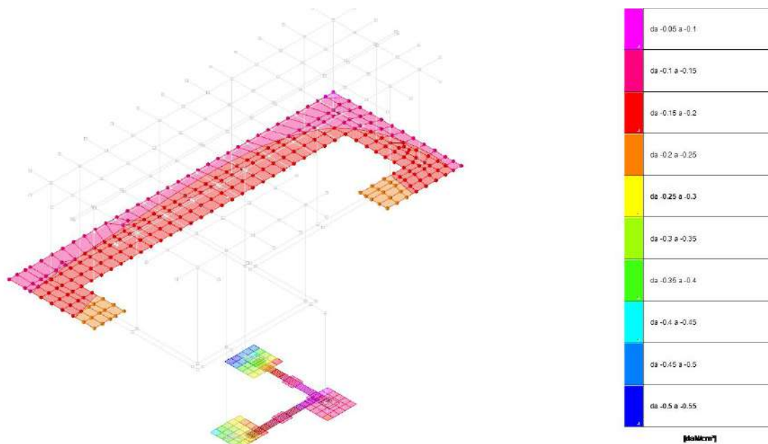
Pressioni massime sul terreno
