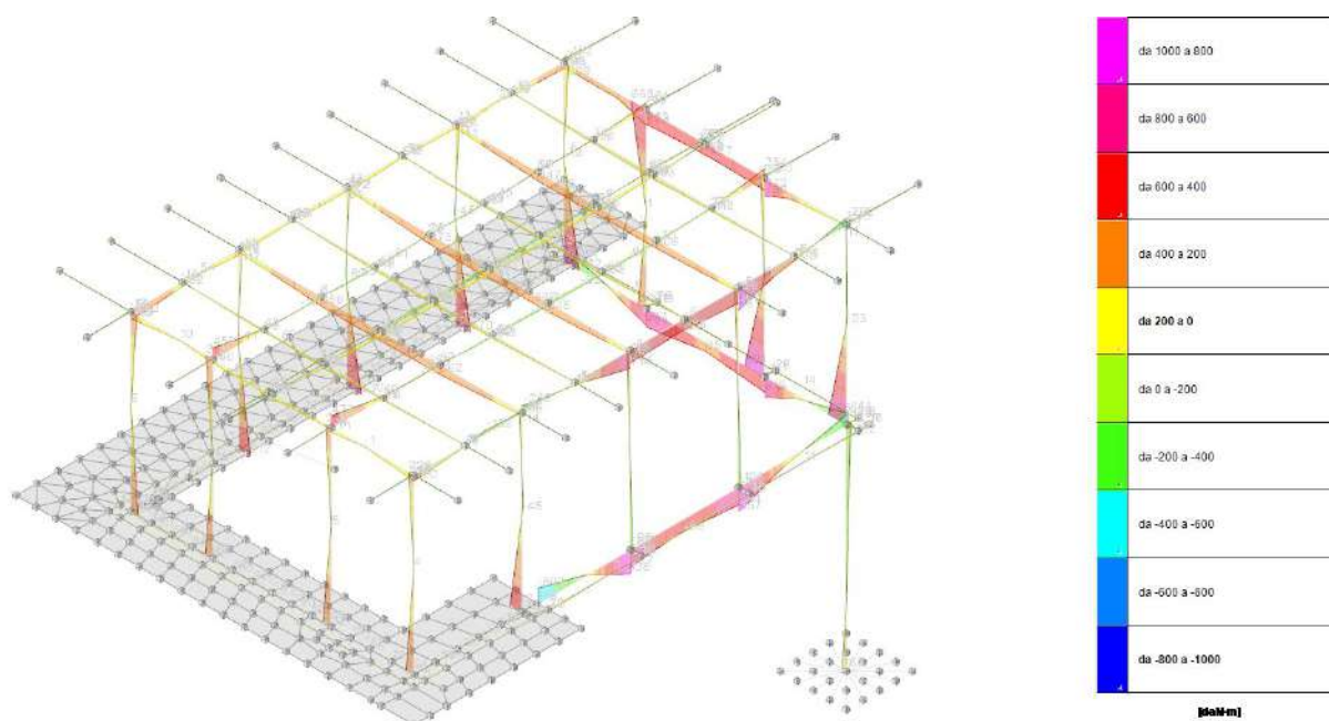
sollecitazioni aste M3 massime
