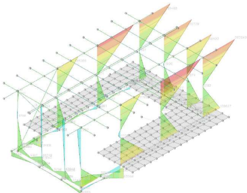
sollecitazioni aste M2 massime
