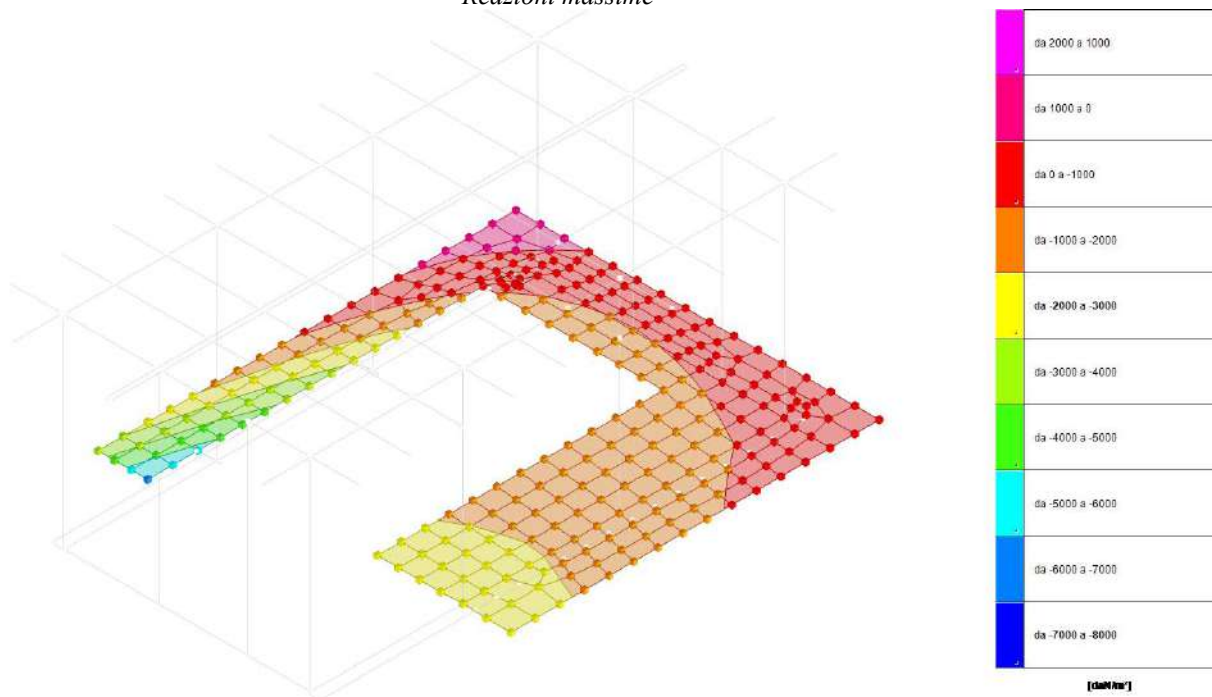
Pressioni massime sul terreno
