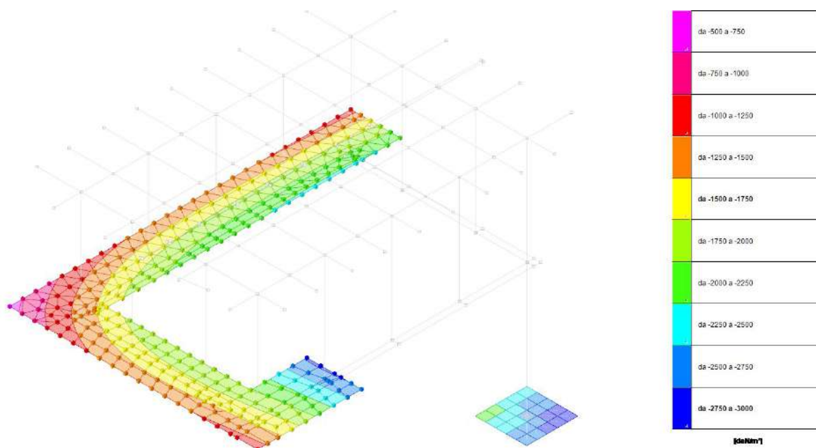
Pressioni massime sul terreno
