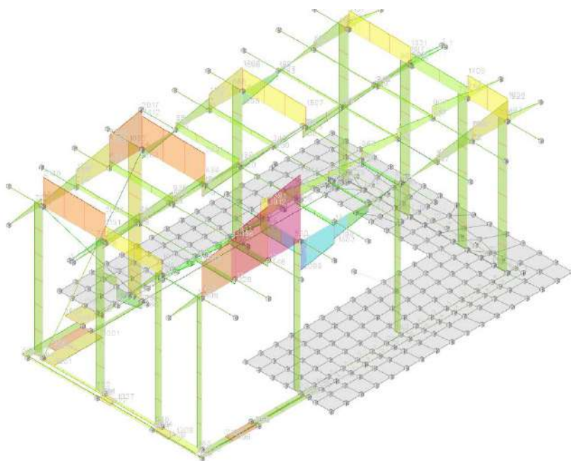
sollecitazioni F2 massime
