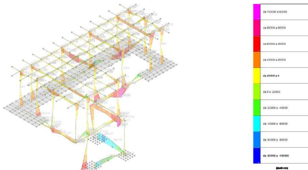
sollecitazioni aste M3 massime
