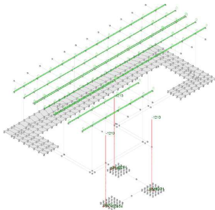
Carichi in Condizione pesi strutturali
