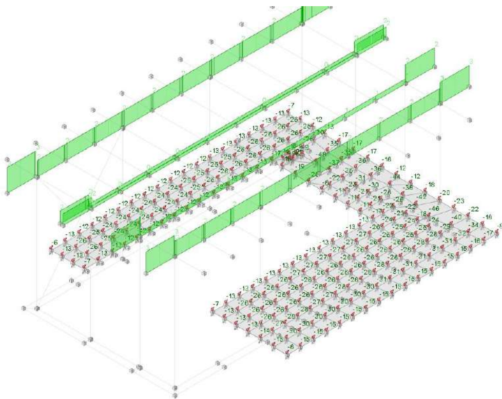
Carichi in Condizione Variabili H
