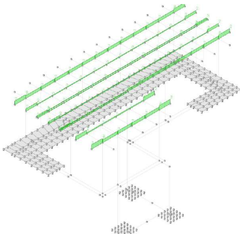
Carichi in Condizione Variabili H
