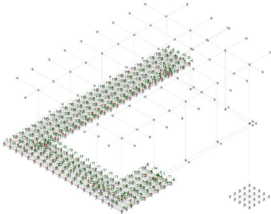
Carichi in Condizione Variabili C
