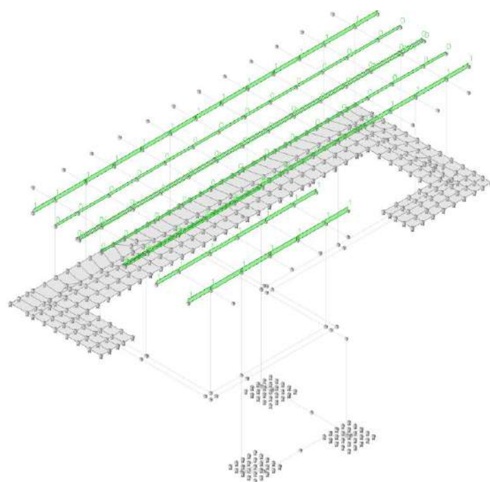
Carichi in Condizione Neve
