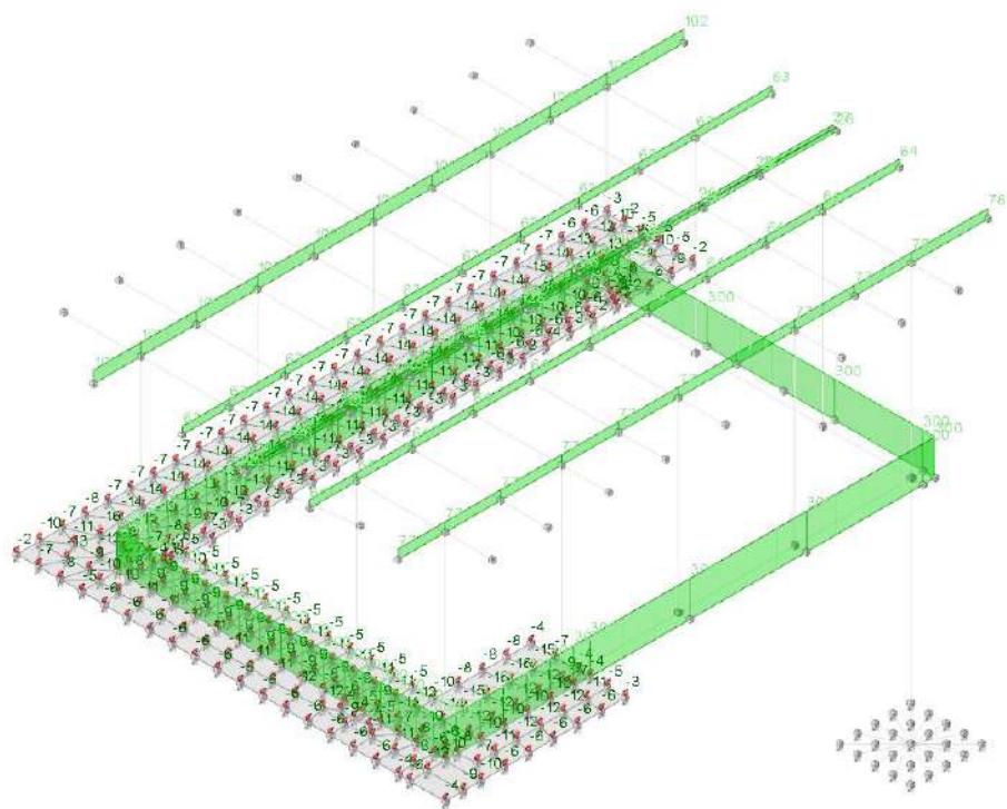
Carichi in Condizione permanenti portati
