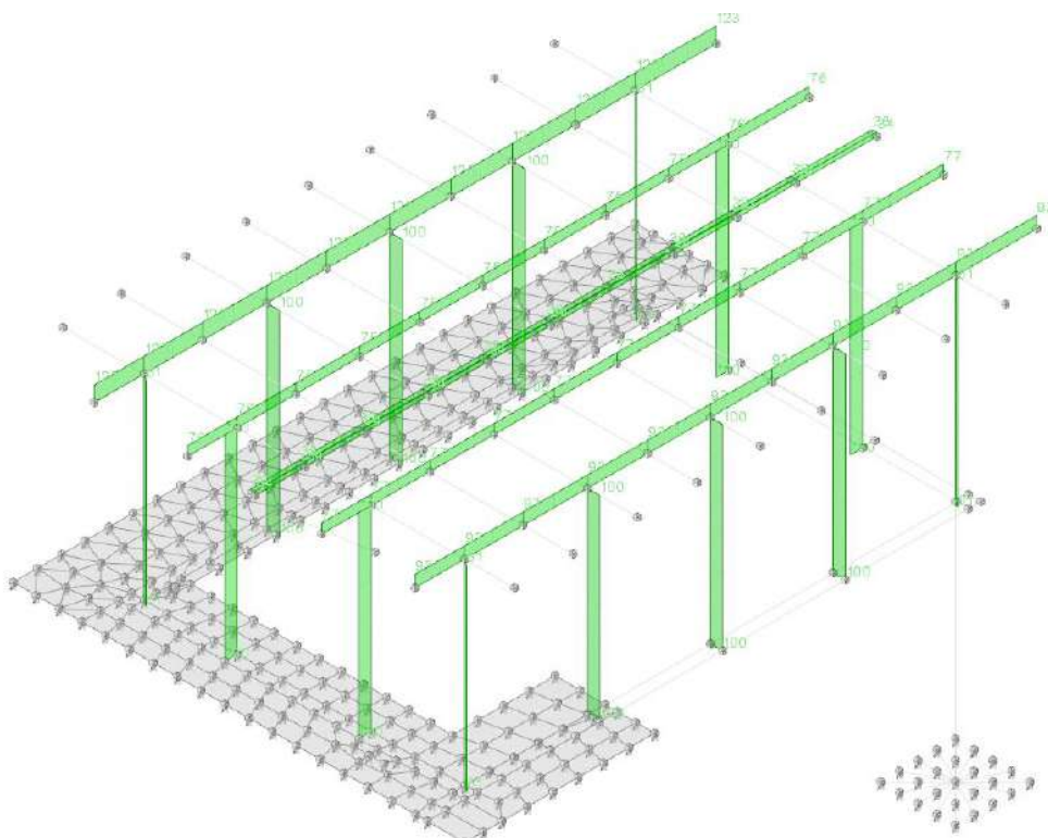
Carichi in Condizione Vento
