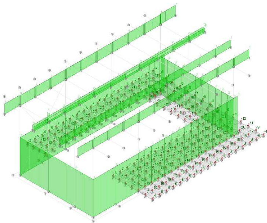
Carichi in Condizione permanenti portati
