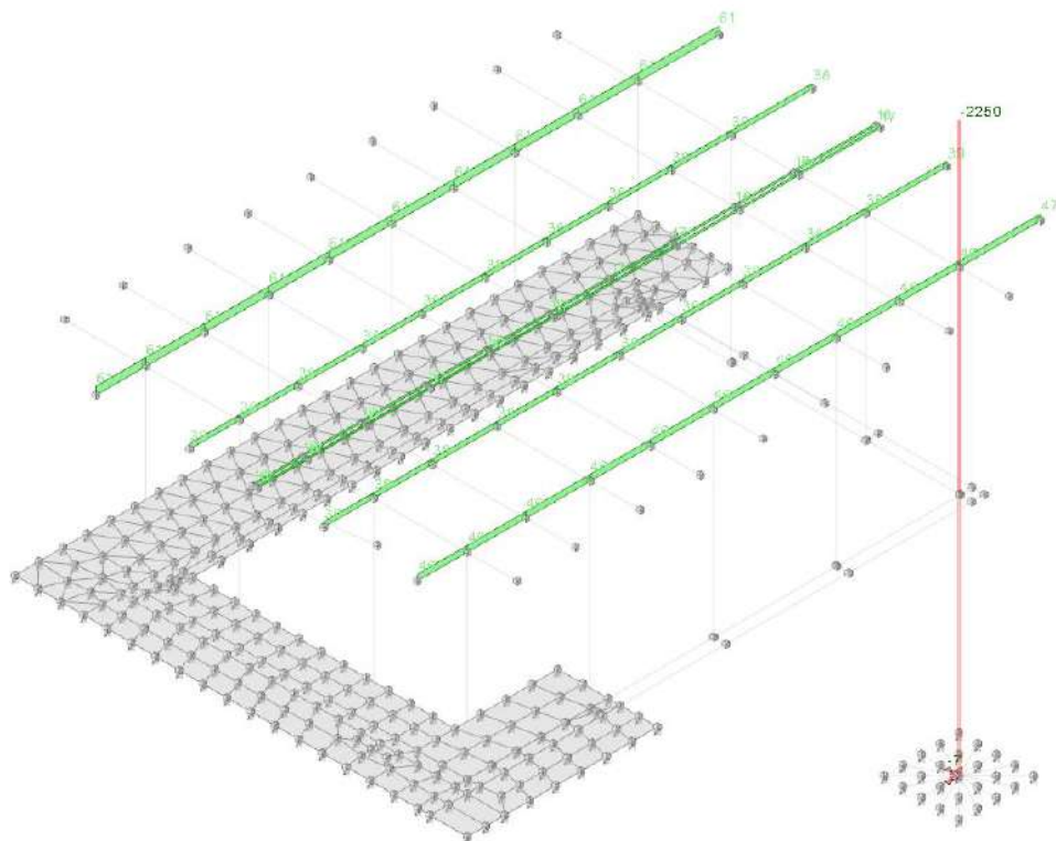
Carichi in Condizione pesi strutturali
