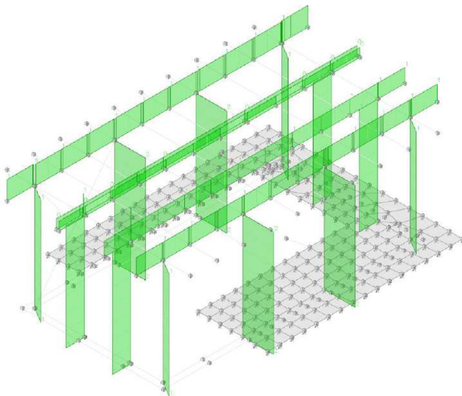
Carichi in Condizione Vento
